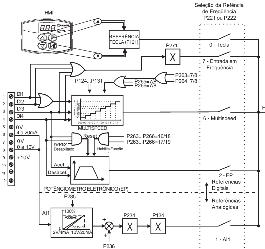
Figura 6.1 - Blocodiagrama da referência de frequência
