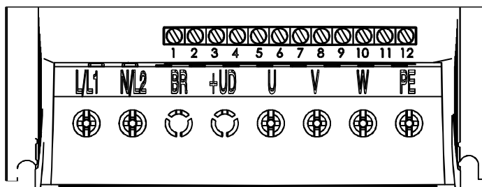
Figura 3.4 a) b) - Bornes da potência
