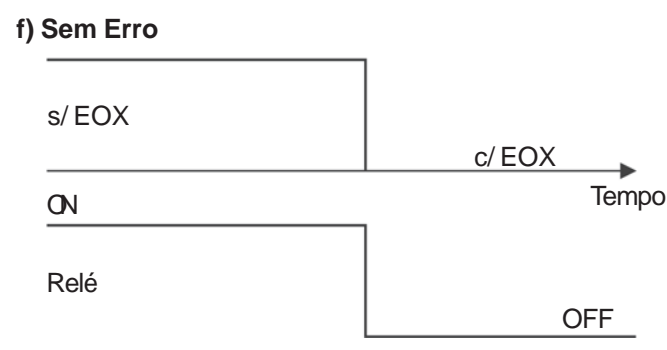
Figura 6.20 a) a f) - Detalhes do funcionamento das funções das saídas digitais
