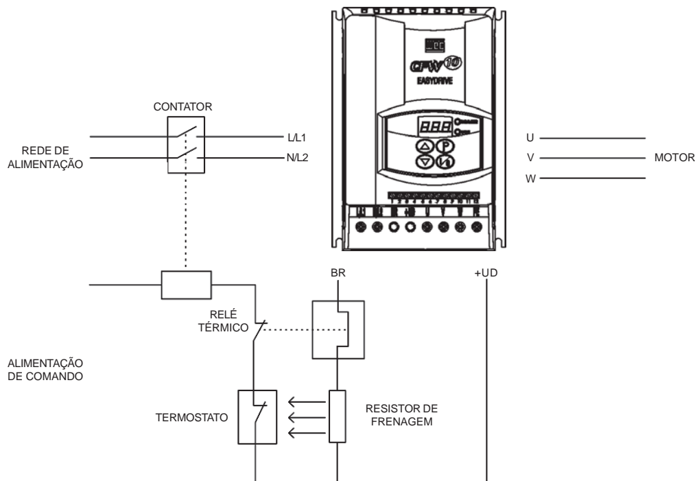
Figura 8.4 - Conexão do resistor de frenagem (só para os modelos 7,3A e 10A/200-240 V e 4,0A/110-127 V)
