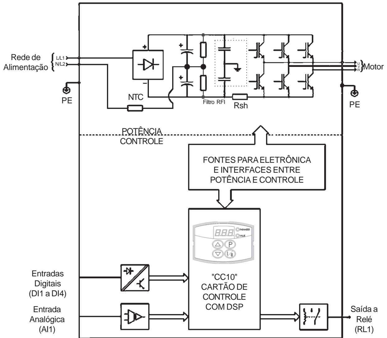
Figura 2.3 - Diagrama de Blocos do CFW-10 modelos 1.6A e 2.6A/110-127V
