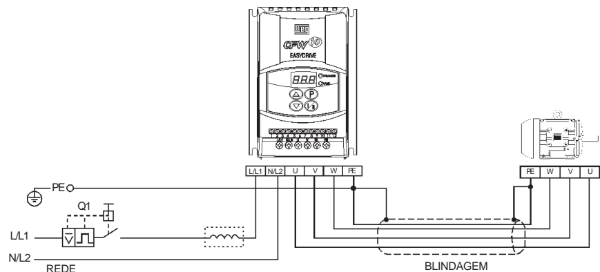
Figura 8.2 - Conexões de potência com reatância de rede na entrada
