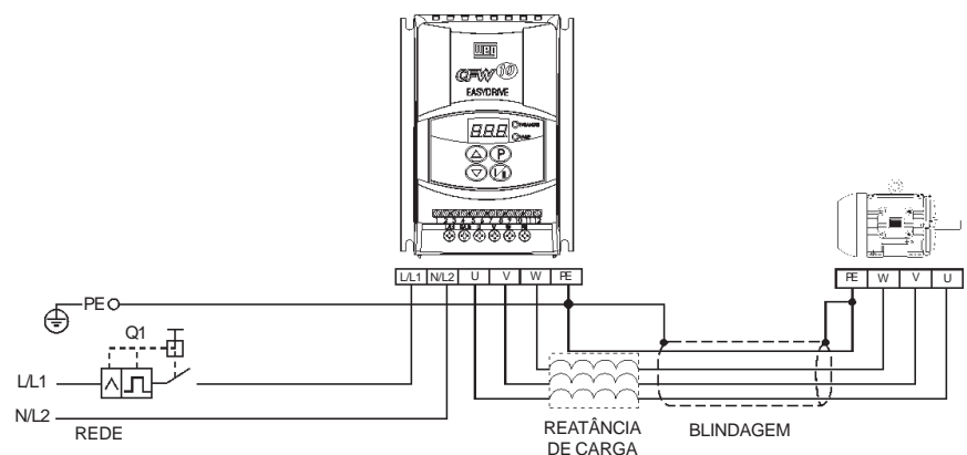
Figura 8.3 - Conexão da reatância de carga
