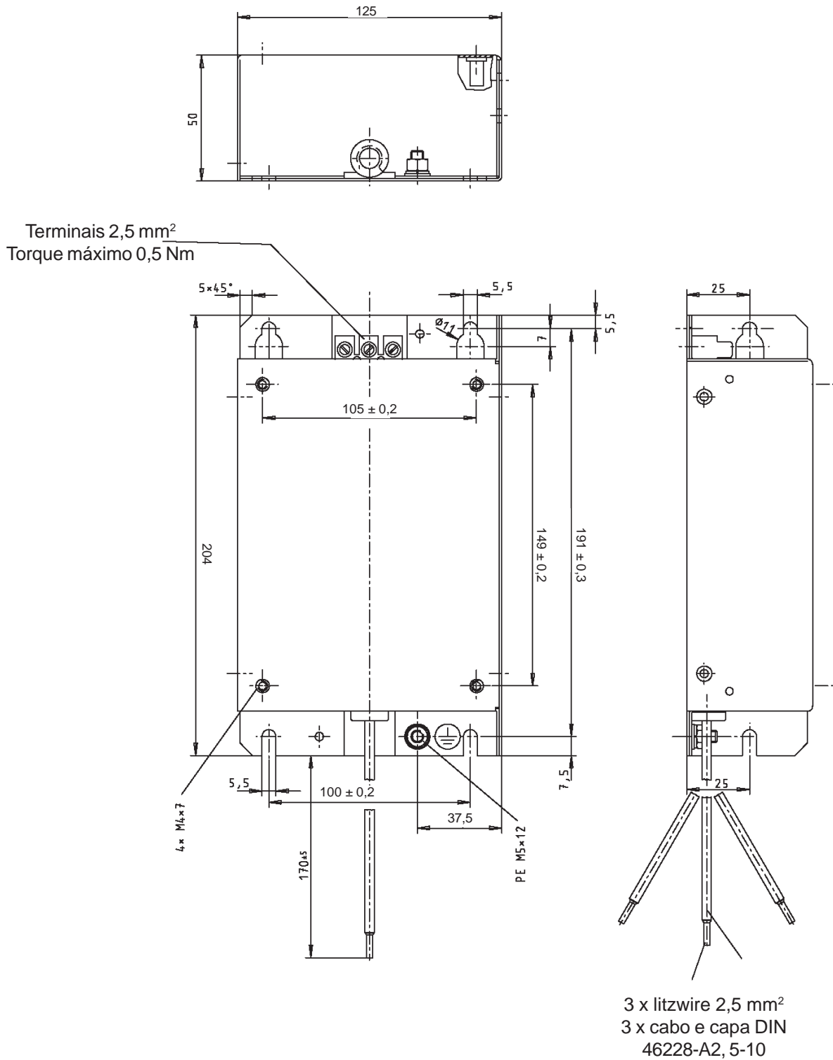
Figura 3.14 b) - Desenhos dos filtros footprint / booksize
