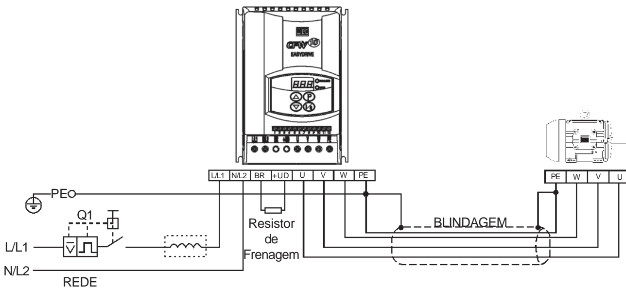
Figura 3.6 a) b) - Conexões de potência e aterramento
