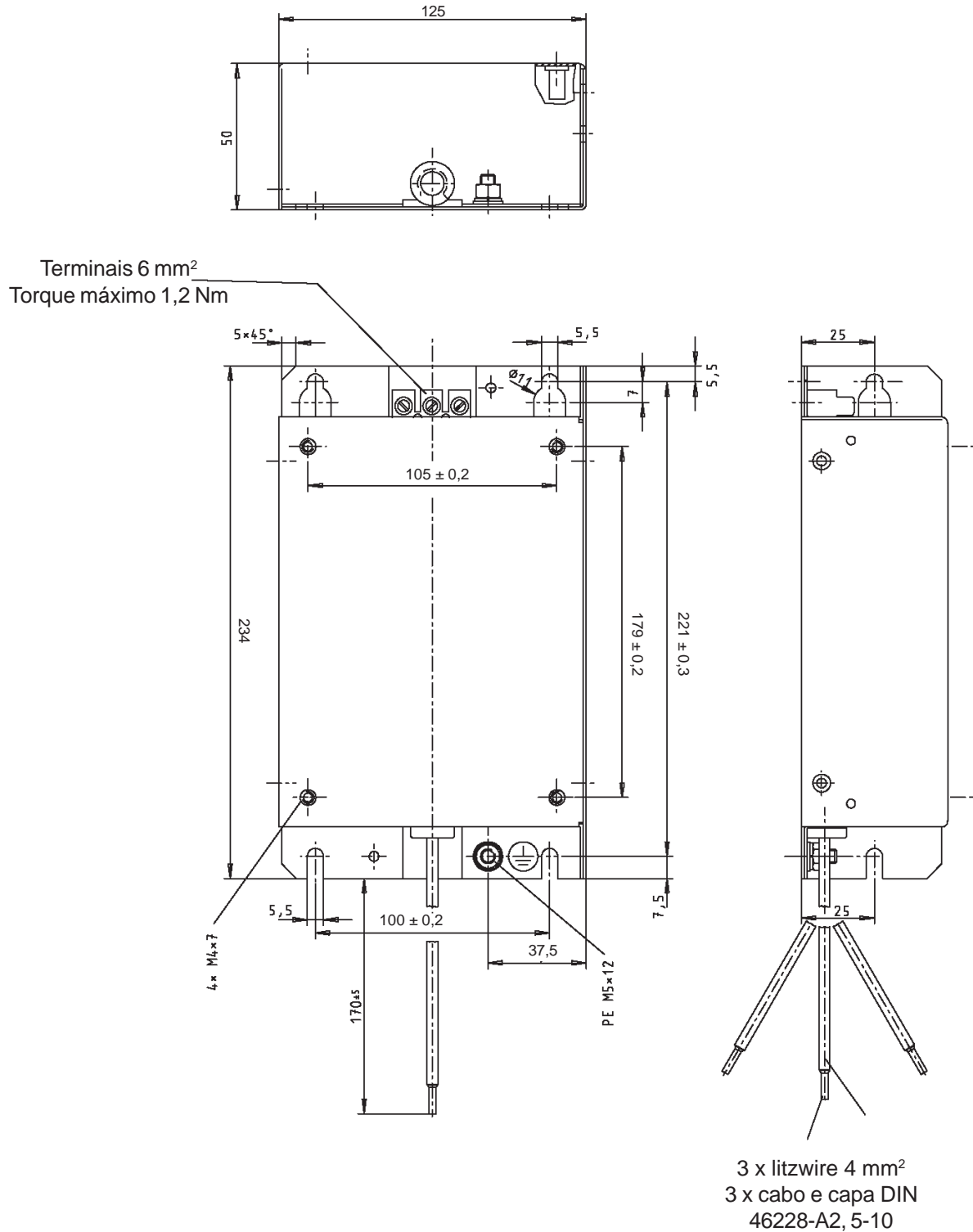
Figura 3.14 c) - Desenhos dos filtros footprint / booksize
