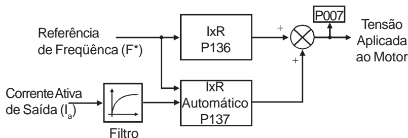
Figura 6.7 - Blocodograma da função boost de torque automático
