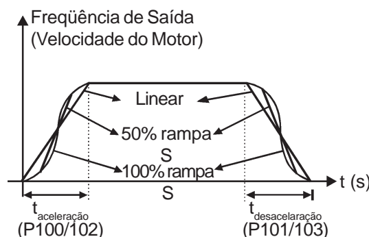
Figura 6.4 - Rampa S ou linear
