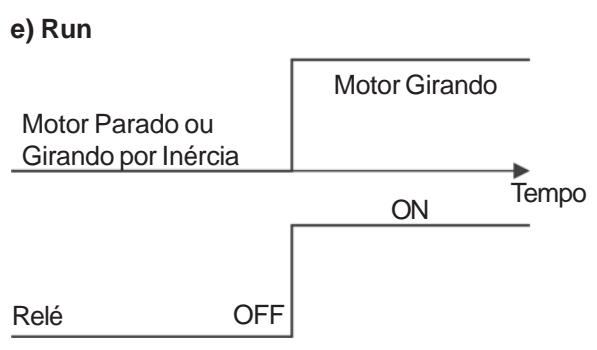
Figura 6.20 a) a f) - Detalhes do funcionamento das funções das saídas digitais
