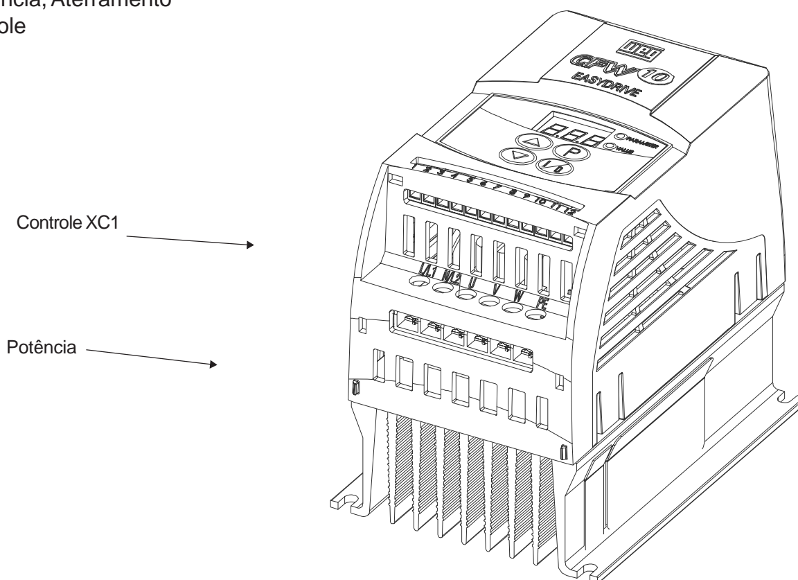
Figura 3.4 a) b) - Bornes da potência
